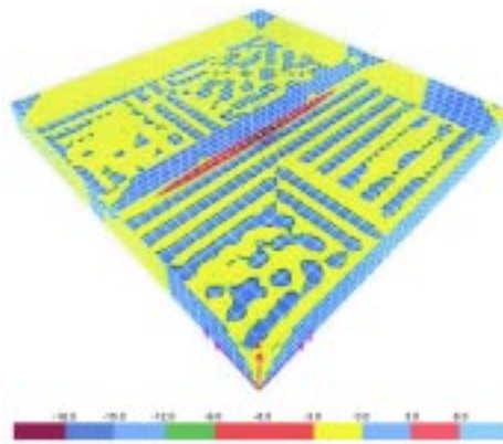
Figura 3 - Diagramas de esforços solicitantes (SAP 2000 – momentos fletores), considerando os recalques previstos
