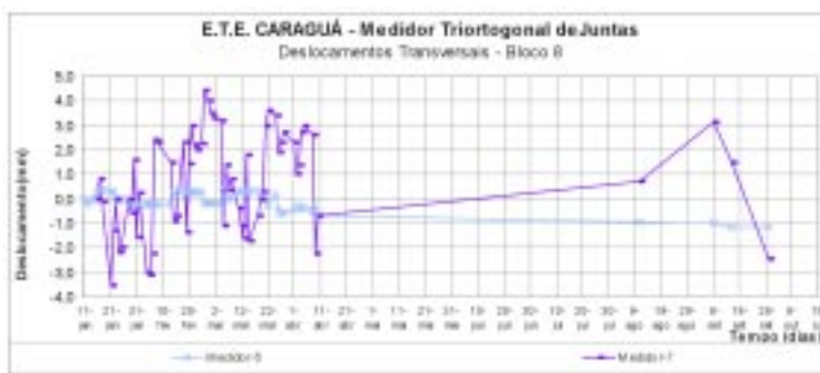
Figura 7 – Gráficos com leituras dos medidores triortogonais (deslocamentos transversais - Bloco 8)
